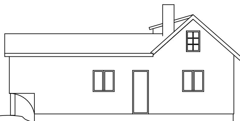
Fasad Väster
