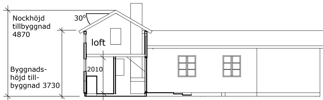
Sektion B-B
