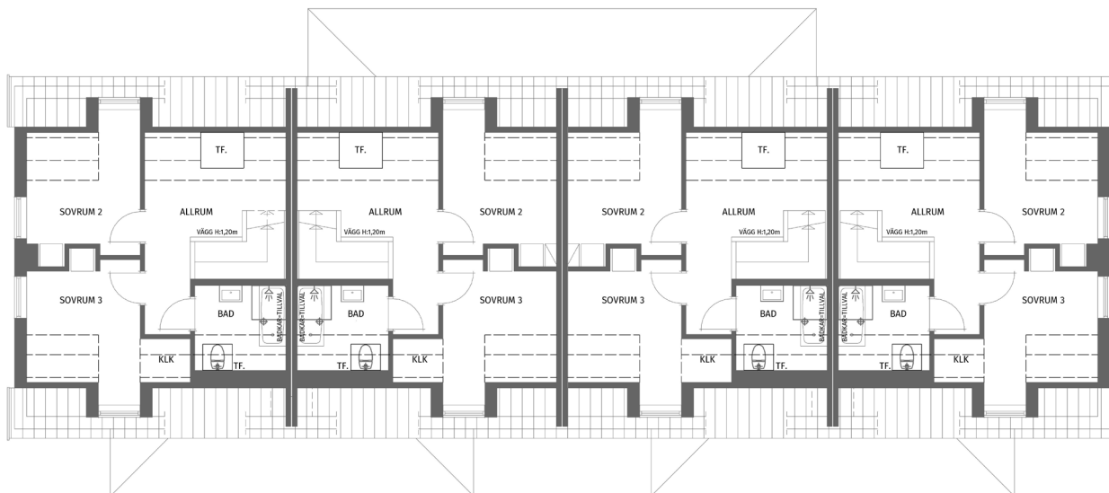
ÖVERVÅNING
