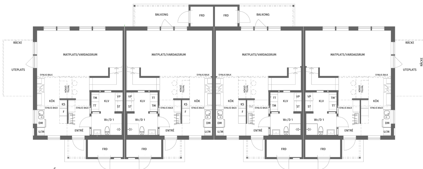
ENTRÉPLAN
